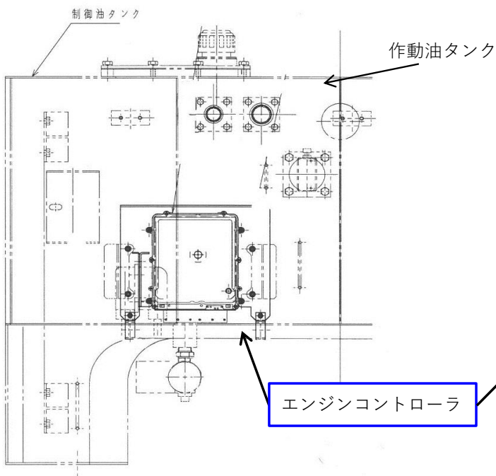
「ニイガタNR303ロータリ除雪車」
